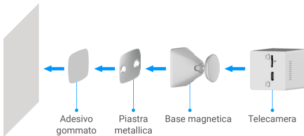
Fig. 1 Montaggio con adesivo gommato
